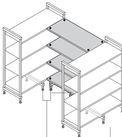
Unidad en forma de U Dos unidades iniciadoras + anaqueles intermedios
