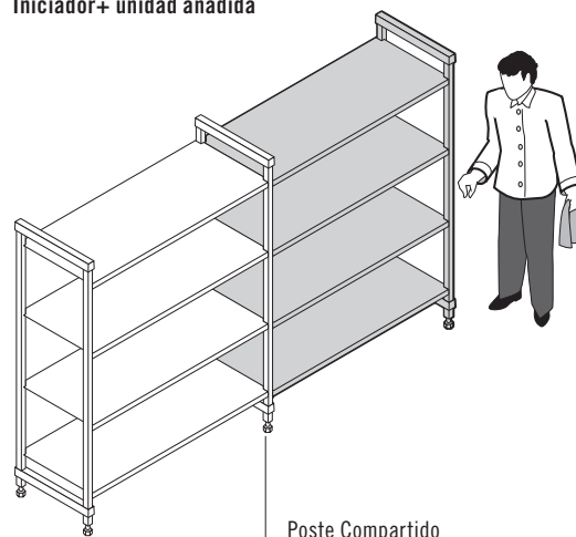
Poste Compartido
